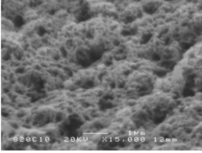
DYO UV nanokompozit SEM fotoğrafı
